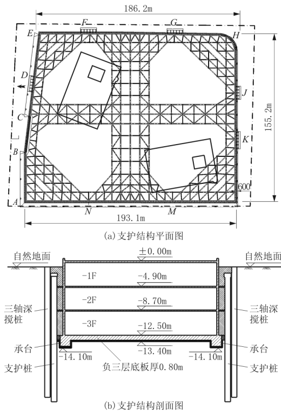
图1 支护结构示意图
