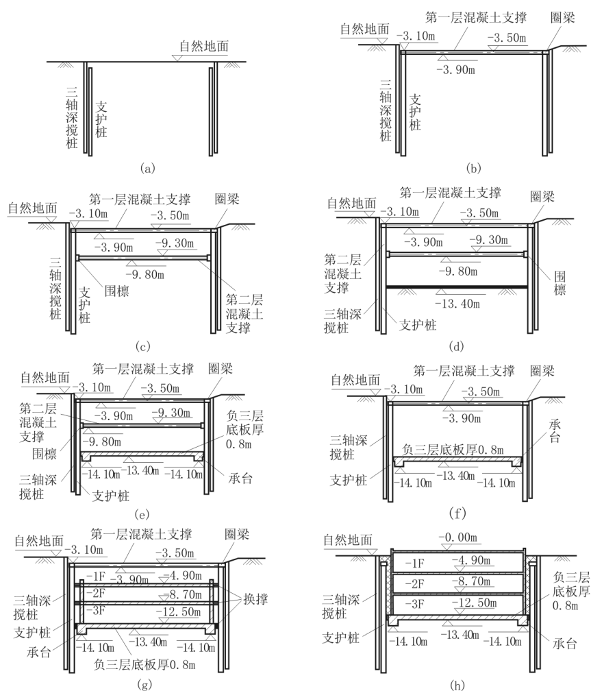
图 3 基坑施工过程
