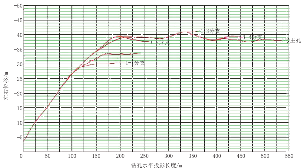
图 3 钻孔轨迹平面图
