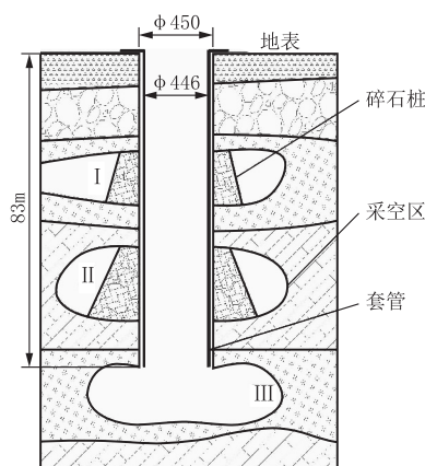
图 1 钻井结构示意图
