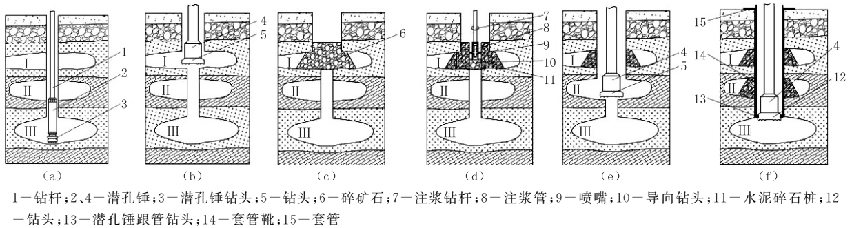
图2 多层采空区成井工艺流程图
