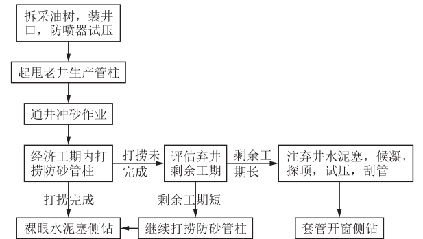
图1 侧钻方案决策图
