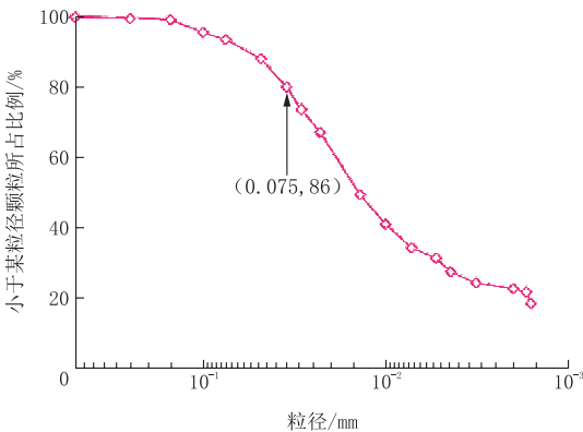
图 1 温州原始泥浆颗粒分曲线
