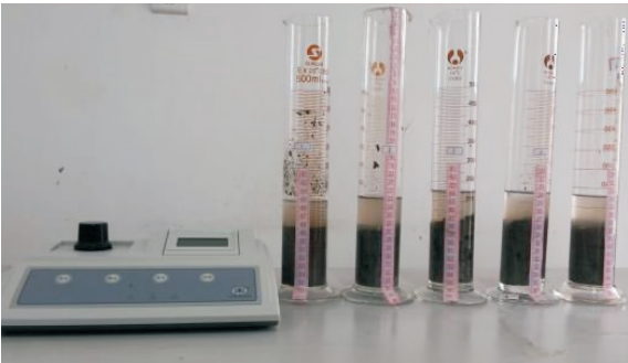
图 2 沉降柱试验
