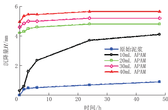
图 3 APAM 沉降量与时间关系曲线
