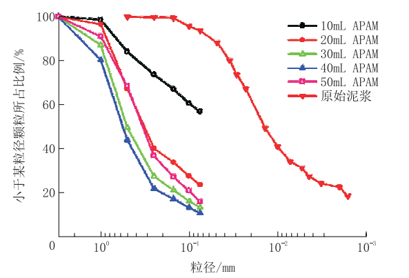
图 8 APAM 颗粒分析曲线
