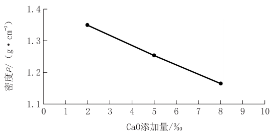
图 6 CaO 絮体密度曲线
