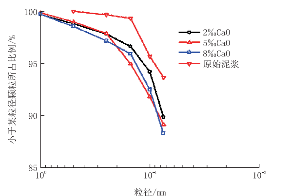
图 9 CaO 颗粒分析曲线
