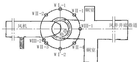
图 1 帷幕注浆施工方案示意
