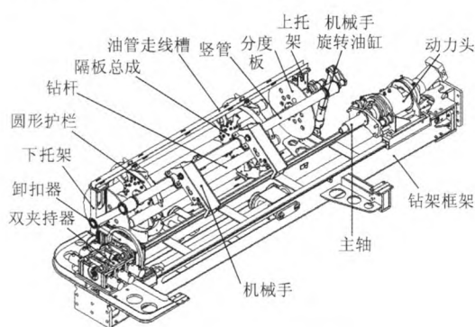
图1 钻杆储管架总体结构图
