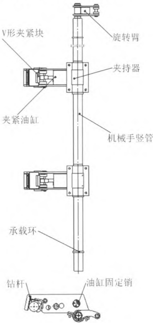
图 6 机械手结构图
