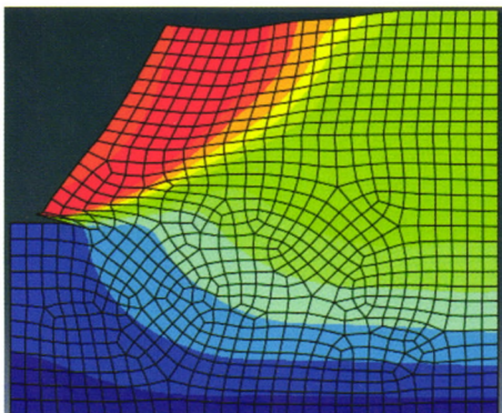
图 4 位移矢量图
