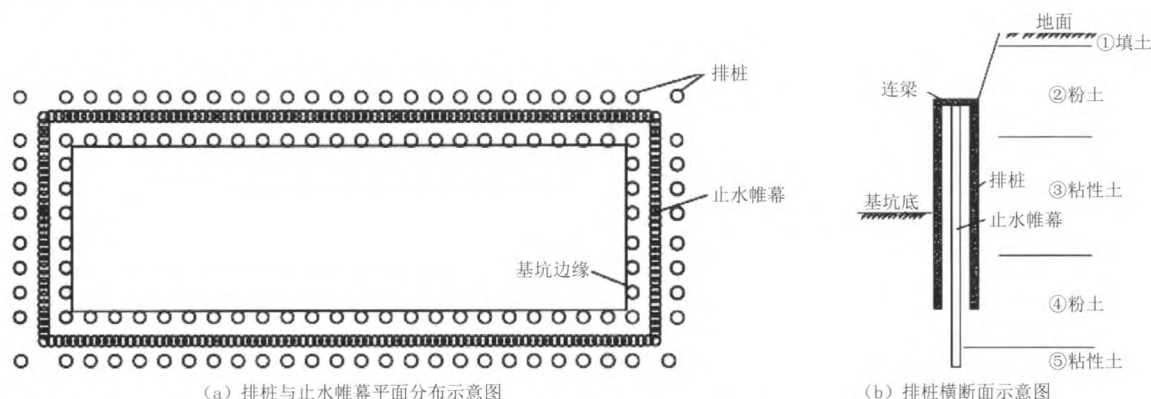
图 1 双排桩支护加水帷幕示意图
