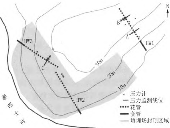
图 8 水平排放孔平面布置图
