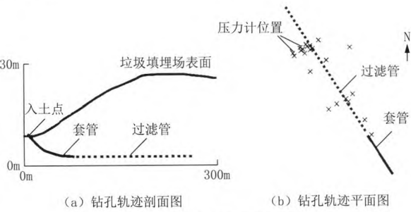
图 6 钻孔轨迹示意图
