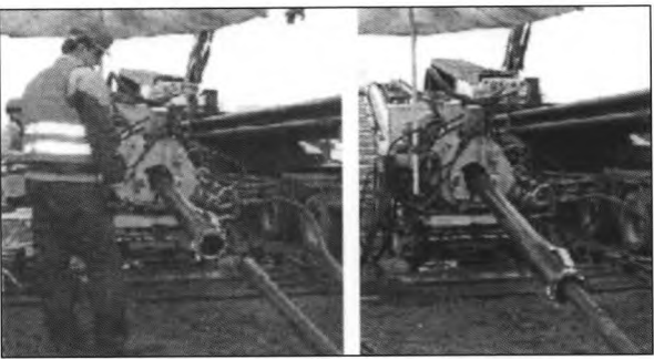
图 7 施工现场
