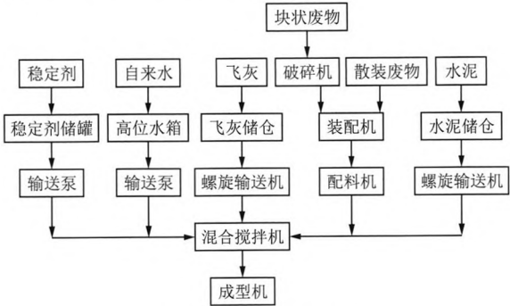
图 3 稳定化/固化工艺流程
