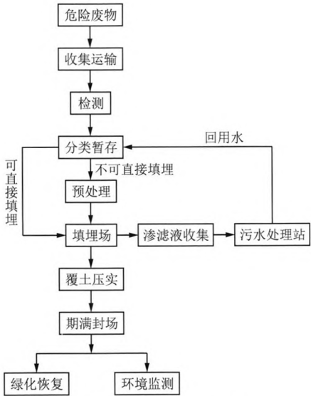
图 2 填埋处置总体工艺流程
