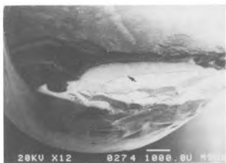
图4 金刚石层由于热损伤与胎体分层
