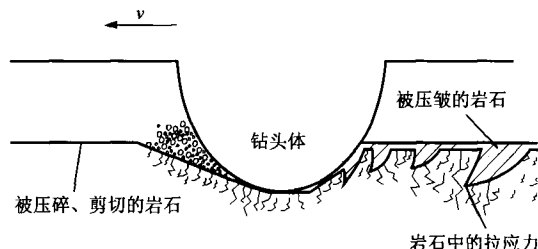
图1 磨粒磨损示意图
