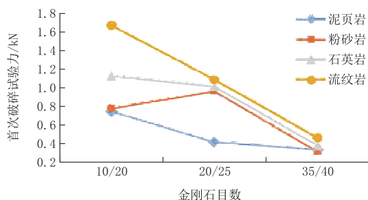
图6 不同金刚石压入岩石首次破碎试验力值变化曲线
