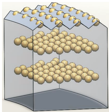
图8 多级金刚石表孕镶钻头14/16目大颗粒金刚石三层布齿结构示意图
