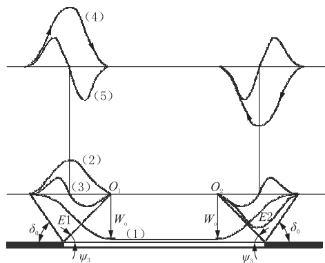
(1)—下沉曲线;(2)—倾斜曲线;(3)—曲率曲线;(4)—水平移动曲线;(5)—水平变形曲线
