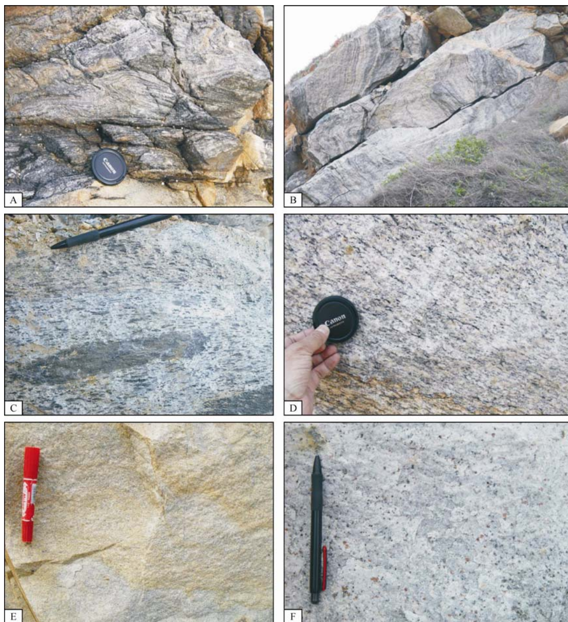
图 14 长乐—南澳构造带发育的早白垩世岩浆岩和变质岩
