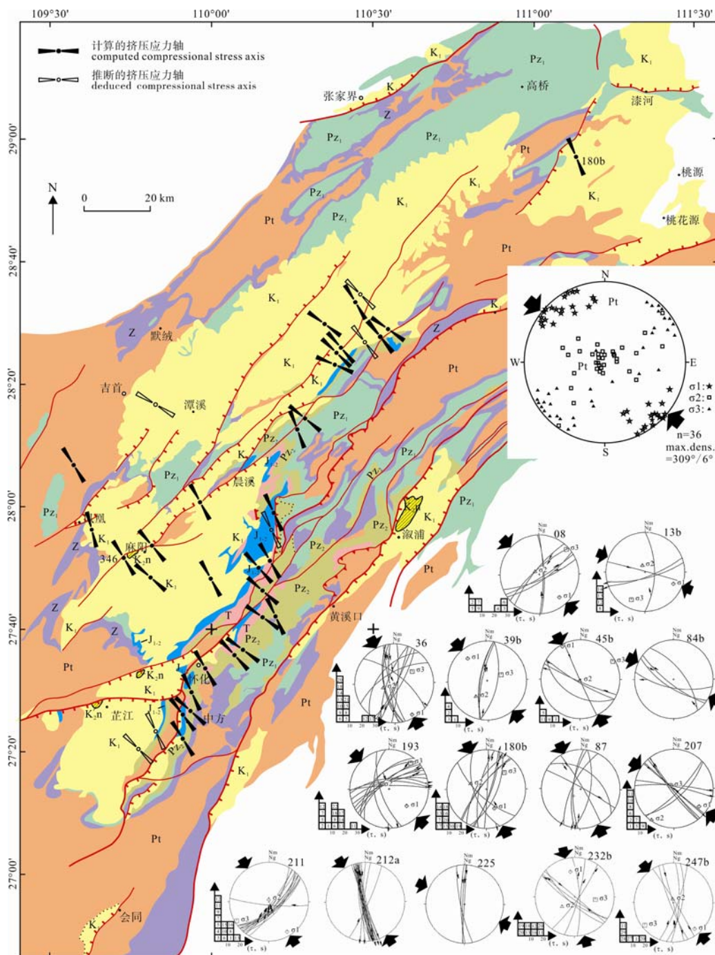
图 5 沅麻盆地早白垩世 NW—SE 向挤压构造应力场
