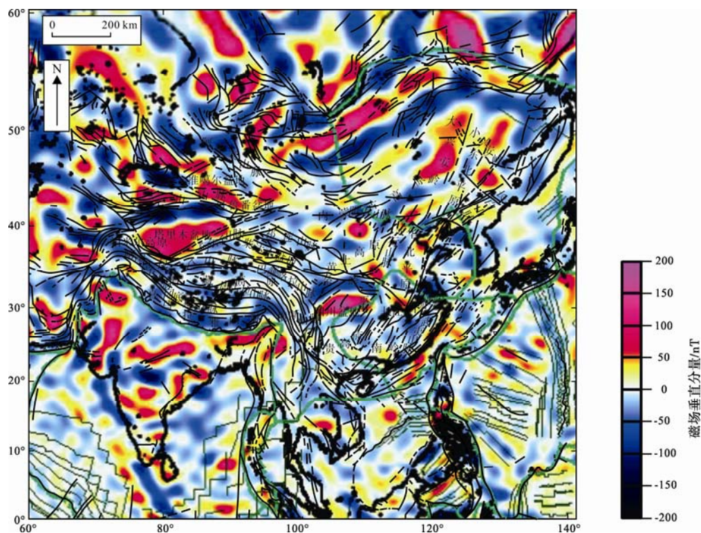
图 2 中国大陆及其邻区地壳磁场垂直分量图(据 Maus et al., 2008; Müller et al., 2008; Abdolazim, 2001 等编制)
