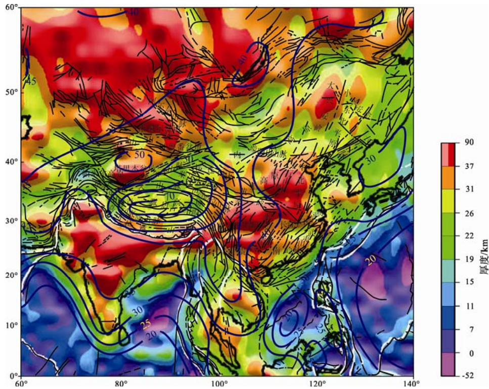
图 3 中国大陆及其邻区磁性地壳厚度图(据 Fox Maule et al., 2005; Abdolazim, 2001 等编制)
