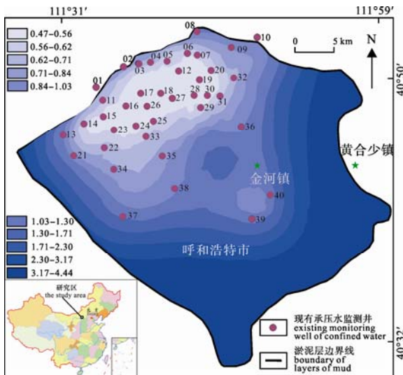
图 2 优化前估计误差标准差等值线图
