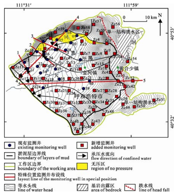
图 3 优化后监测井分布图
