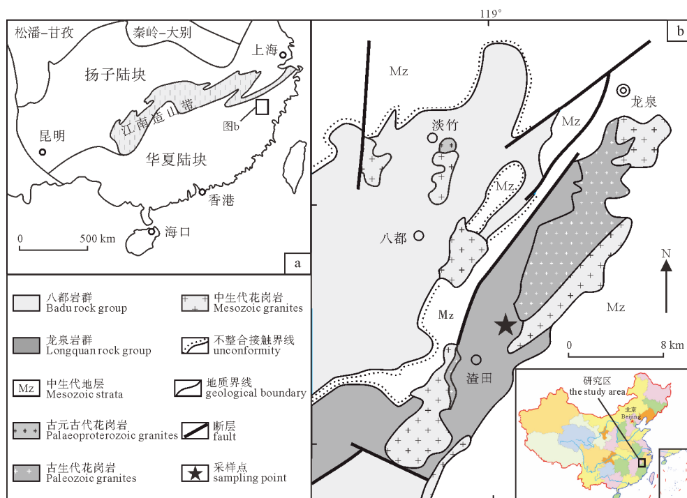
图1 研究区大地构造位置(a)、龙泉地区地质简图(b)(据 Xing et al., 2014 修改)
