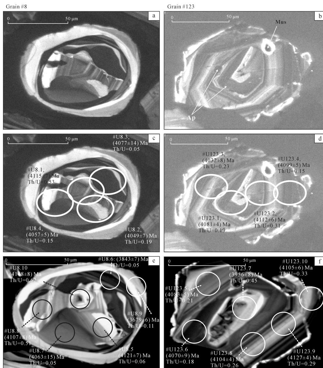
图2 冥古宙锆石 CL 图像(据 Xing et al., 2014 修改)
