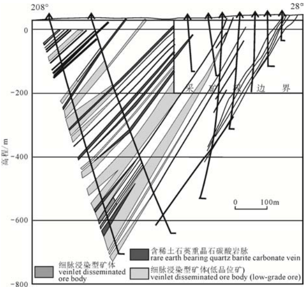
图 6 郝山地区第 5 勘查线剖面 Fig. 6 Section of the 5 th exploration line in Xishan area
