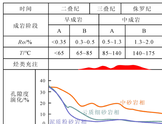
图 4 不同岩相岩石孔隙度演化曲线
