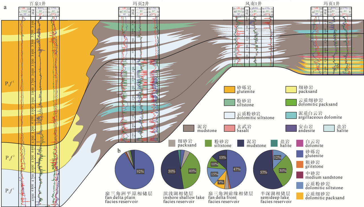
a—岩相剖面图; b—沉积相与岩相展布统计关系。
