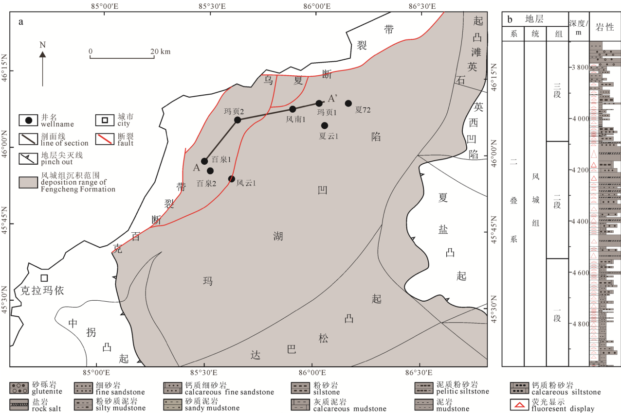
图 1 玛湖凹陷区域构造位置图(a)及玛湖凹陷二叠系风城组地层柱状图(b)
