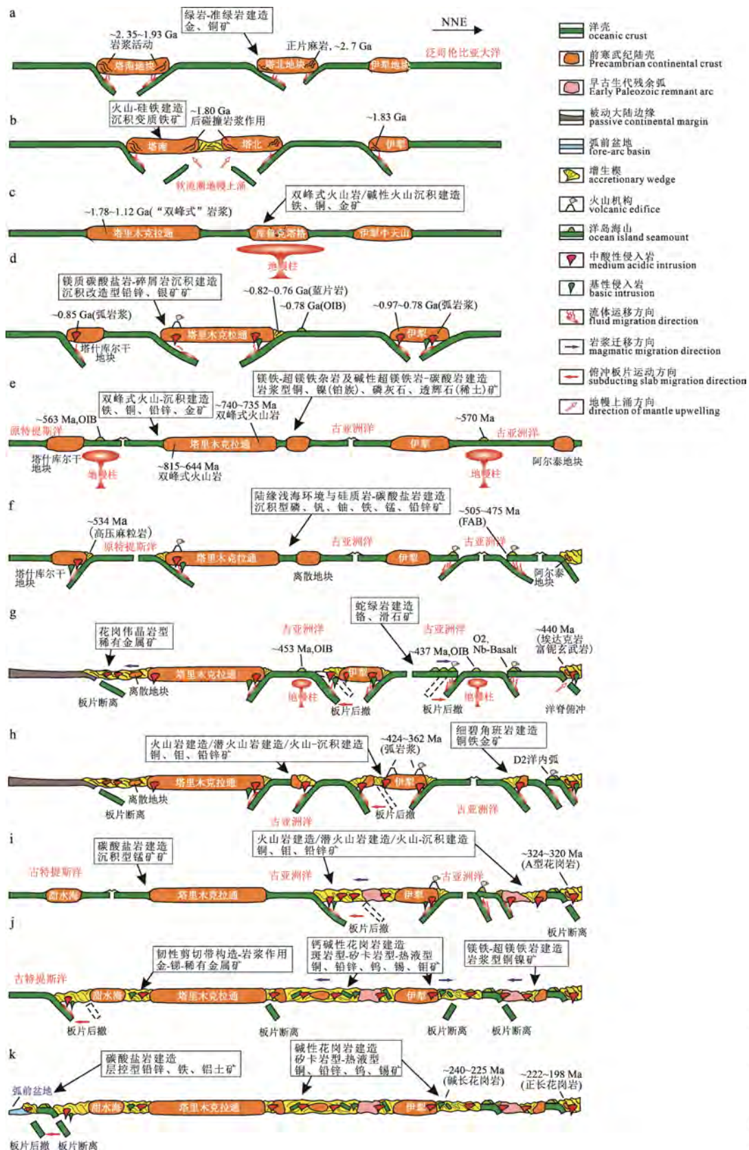
a—太古宙—古元古代; b—古元古代晚期; c—中元古代; d—新元古代早中期; e—新元古代晚期; f—寒武纪—早奥陶世; g—中奥陶世—中志留世; h—晚志留世—晚泥盆世; i—石炭纪; j—早二叠世—早三叠世; k—中晚三叠世。
