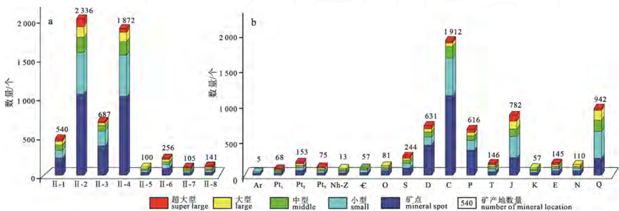
a—成矿省矿床点分布; b—各地质时代矿床点分布。
