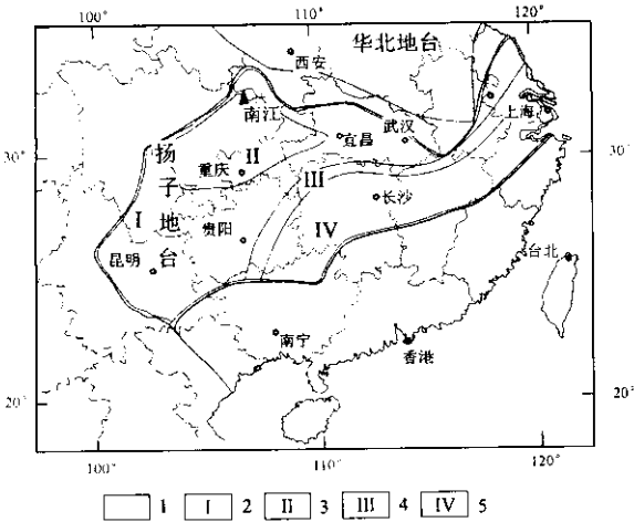
图1 区域地质图(据 Steiner 等,2001 有改动)
