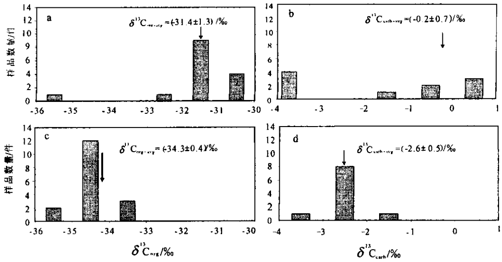
图 3 下寒武统郭家坝组 C 同位素组成比较 Fig. 3 Carbon isotope composition distribution of the study in the Guojiaba Fm. a,b-郭家坝组上部 ;c,d-郭家坝组下部 a,b-upper of Guojiaba Fm. ;c,d-lower of Guojiaba Fm.
