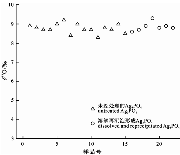
图 3 未经处理的 Ag 3 PO 4 与将其溶解再沉淀形成 Ag 3 PO 4 之间 δ 18 O 测量值的比较 Fig. 3 Comparison in δ 18 O between untreated Ag 3 PO 4 and dissolved and reprecipitated Ag 3 PO 4
