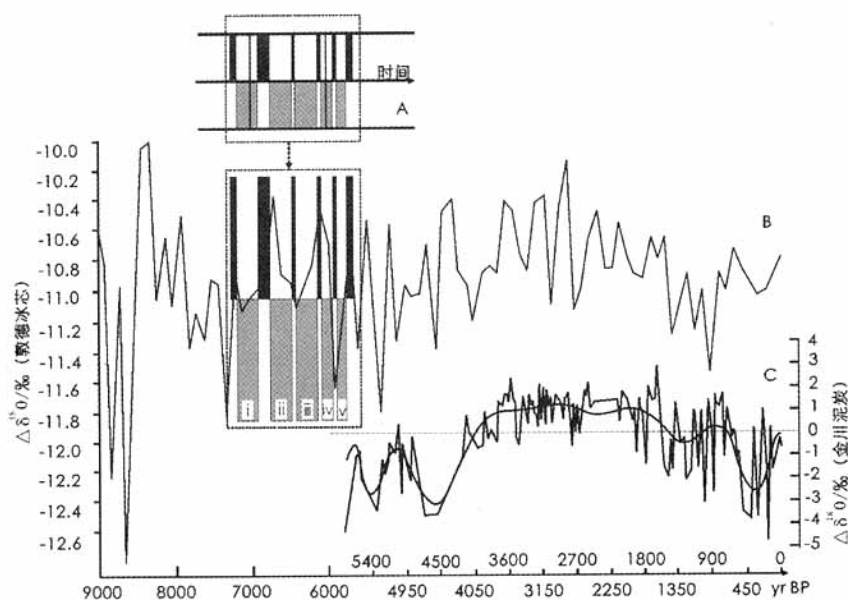
图 3 大吴庄礁体内正常建礁层、水平夹层时空分布与地区性气候变化曲线对比图
