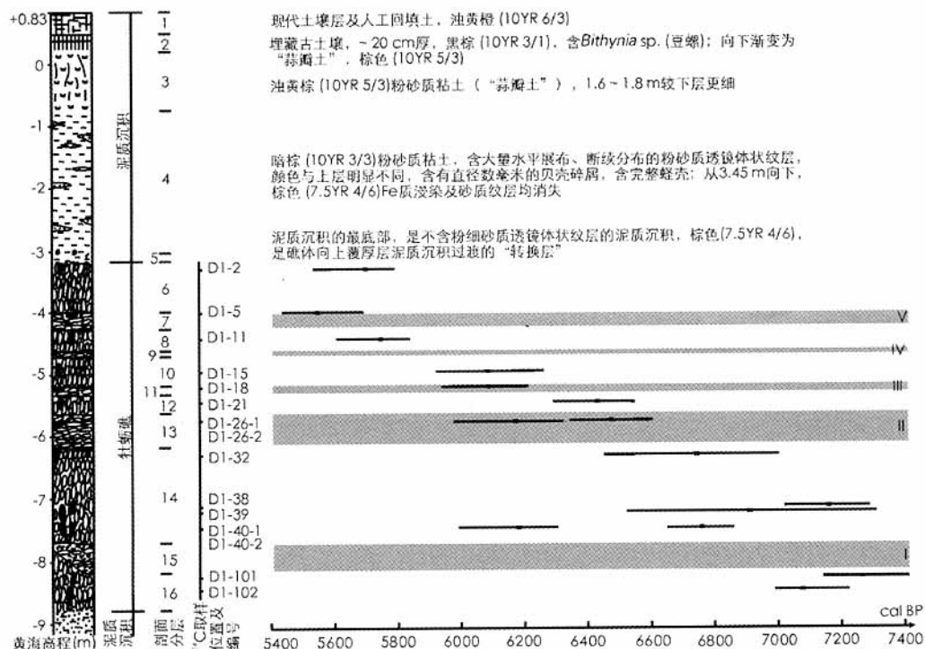
图 2 大吴庄牡蛎礁剖面 1 的地层、 ^{14}\text{C} 取样位置及校正年龄时间—深度分布图
