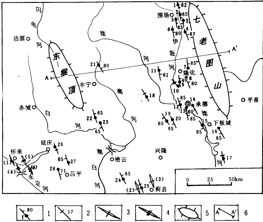
图 1 燕山昌平围地区 NNW 向活动构造形迹图
