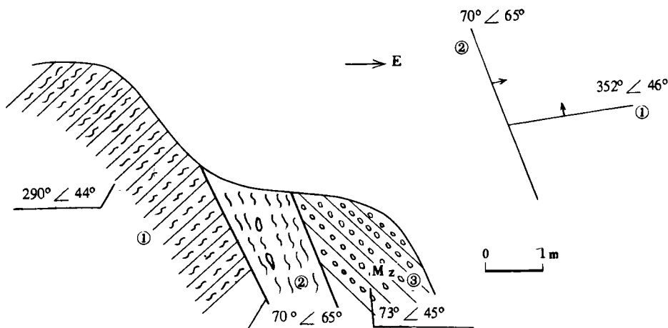
图 5 前双梁垭口南端活动断裂剖面图
