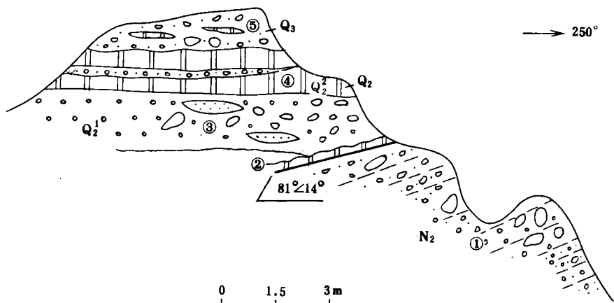
图 7 南口虎峪村新生界地质剖面图
