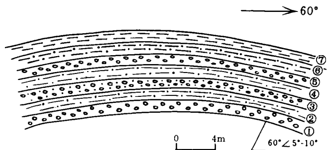
图 8 延庆卧牛山更新统背斜构造剖面图
