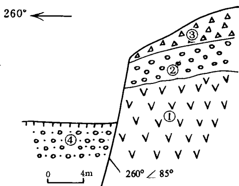
图 3 围场东钓鱼台水库活动断裂剖面图
