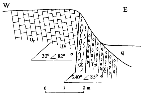
图 4 下板城东良杖子活动断裂剖面图
