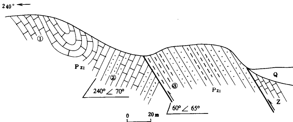
图 6 赵家岭二十里长山活动断裂剖面图
