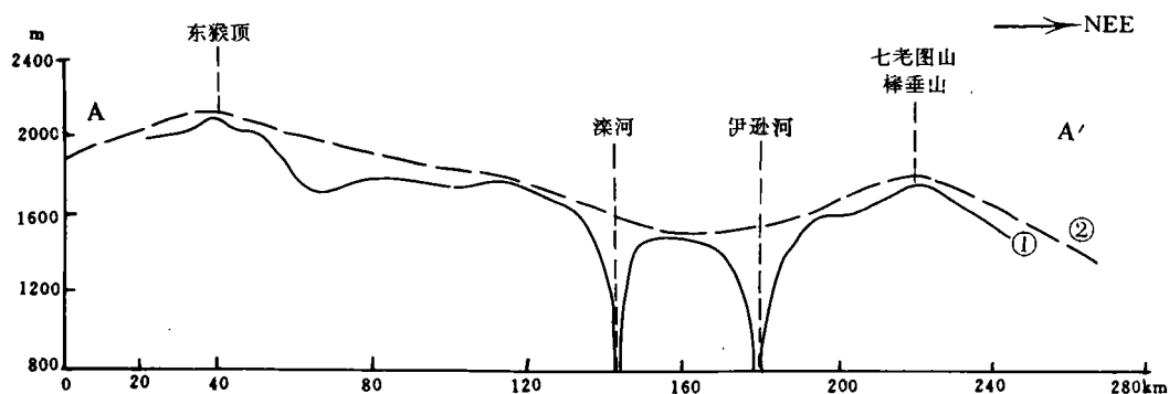
图 9 东猴顶—棒垂山北台期夷平面形变剖面图
