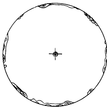
图 3 云母石英片岩中石英光轴等密线图(0—0.5—1—2)
