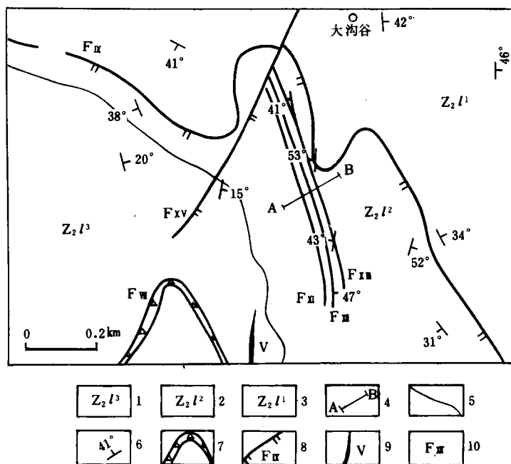
图 1 粤北大沟谷地区地质构造简图
