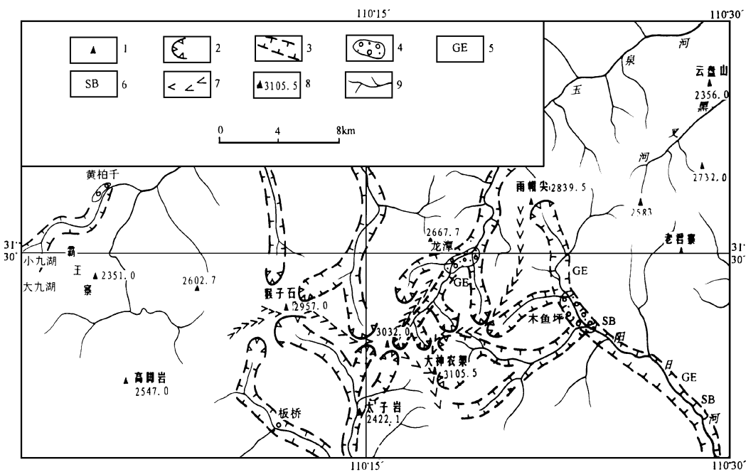
图 1 神农架地区第四纪冰川遗迹分布
