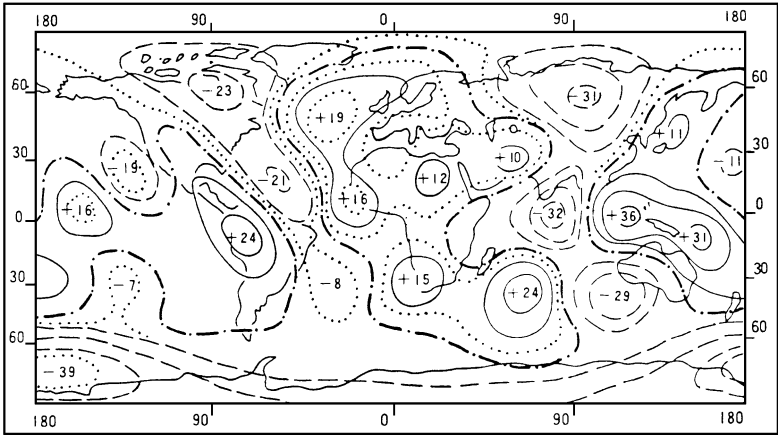
图 2 全球人造卫星重力异常图(据 K Shimazak, 1974 年资料简化)
