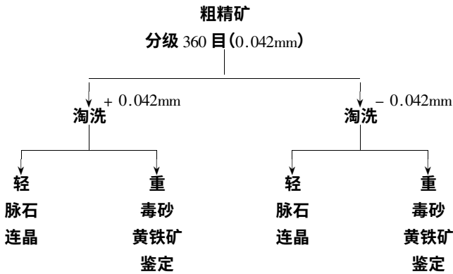
图 2 金属硫化矿物精选提纯流程
