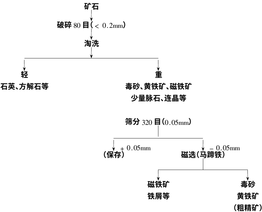
图 1 金属硫化物粗选富集流程
