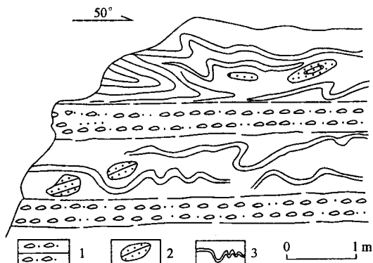
图 4 泥质粉砂岩中的冻融褶皱
