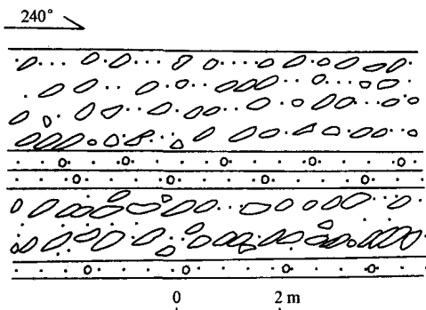
图 3 砾石叠瓦状定向分布示意图
