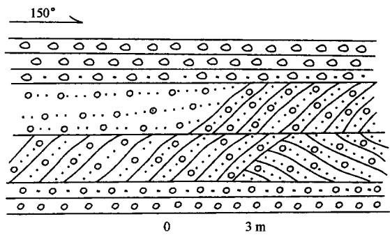
图 2 板状交错层理素描
