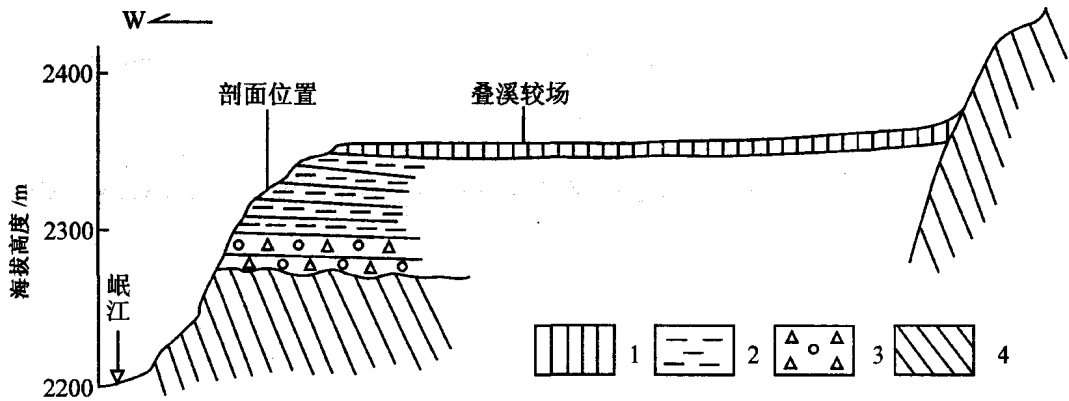
图 2 茂县较场湖相台地横剖面示意图
