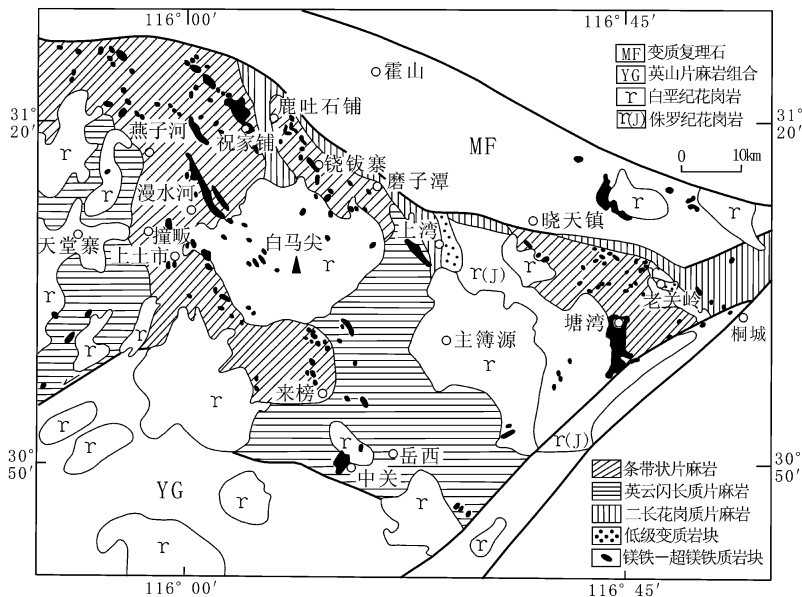
图 3 大别山北部条带状片麻岩组合内镁铁—超镁铁质岩块分布略图 ①
