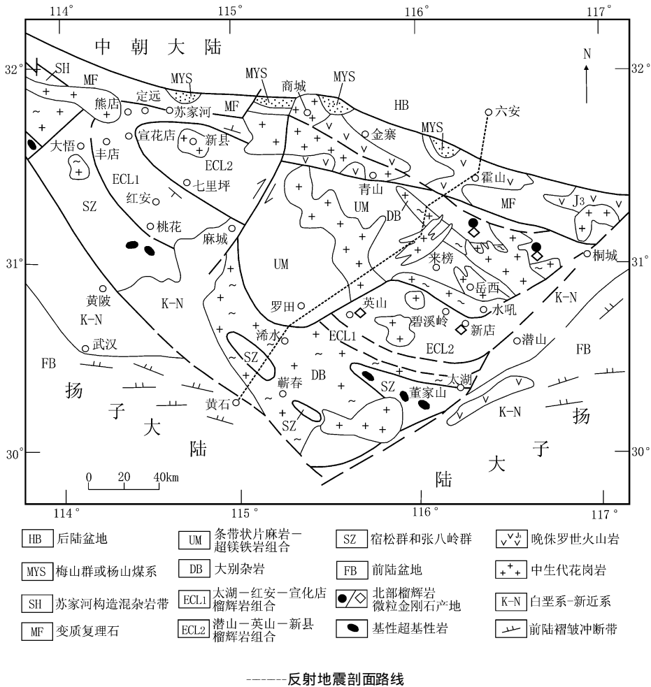
图 1 大别山地质略图
