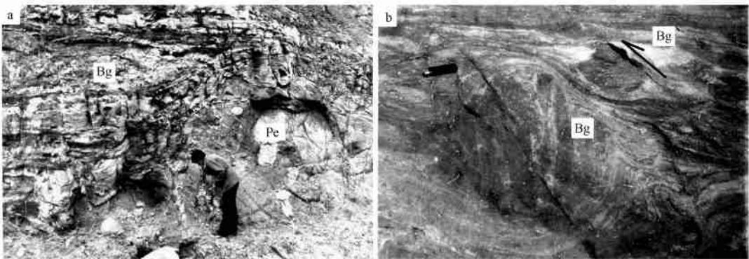
图 2 大别山北部条带状片麻岩中的构造侵位岩块
