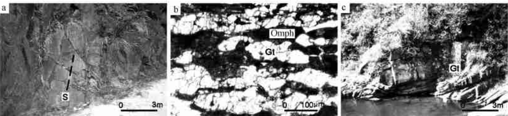
图 8 双河条带状榴辉岩（榴辉岩相糜棱岩）
