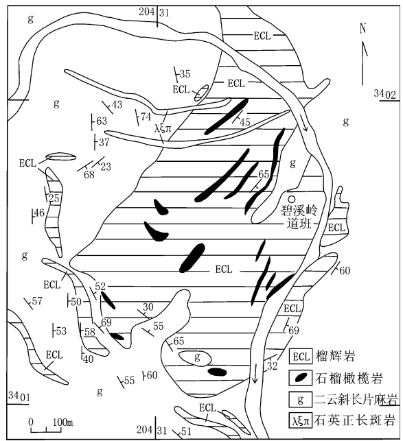
图 7 碧溪岭杂岩体地质略图
