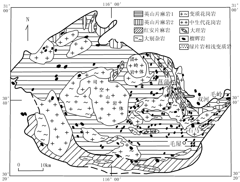
图 6 榴辉岩组合中岩块分布的地质略图
