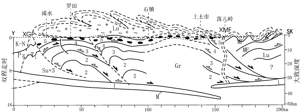
图 15 大别山黄石至六安的偏移反射地震剖面地质解释 (据徐树桐等 2008) [7]
