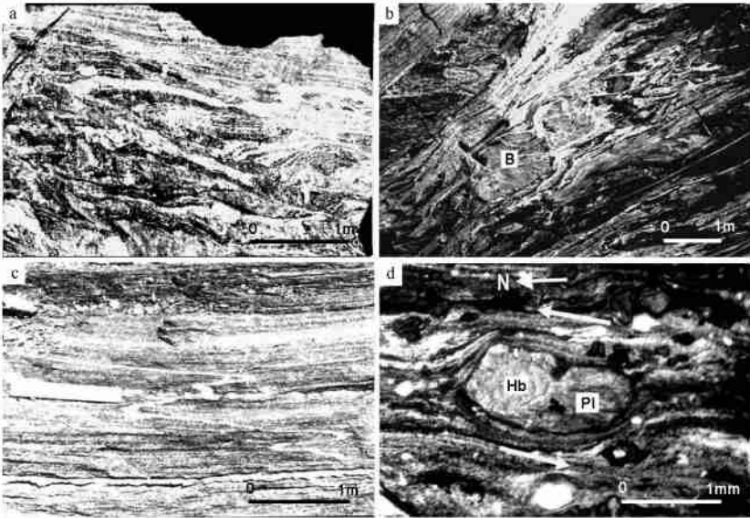
图 5 条带状片麻岩组合内由强烈的剪切造成的糜棱岩
