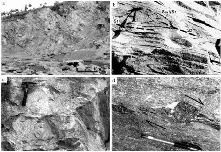
图 13 太湖县石马、石霞、毛屋一带，糜棱岩化并强烈褶皱的榴辉岩相副片麻岩 Fig 13 Mylonitized and strongly folded eclogite paragneiss in the area of Shima, Shixia and Maowu, Taihu County a: 石霞附近斜长角闪质糜棱岩的露头；b: 石霞附近角闪斜长质片麻岩中的重褶；c: 石马东南 糜棱岩化钙硅酸盐岩中的 A 褶皱；d: 毛屋以南英云闪长质糜棱岩中“δ”状榴辉岩块。S m /S 1 : 早期糜棱面理/早起褶皱轴面面理；S 2 : 第二期褶皱的轴面面理。箭头表示运动方向。
