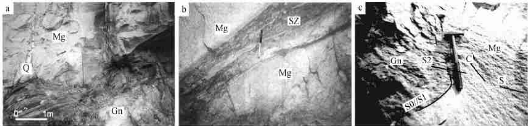
图 12 碱性变质花岗岩露头照片
