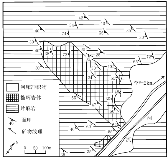
图 10 朱家冲榴辉岩地质图
