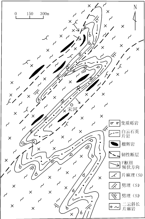
图 11 大别山菖蒲镇宋河村附近浅变质岩片地质略图 [38]
