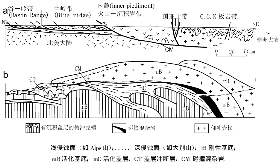
图 14 碰撞造山带的几何结构 (碰撞混杂岩组合的分布) 略图
