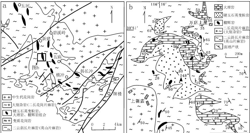
图 9 榴辉岩组合中的大理岩—硬玉石英变粒岩序列分布图
