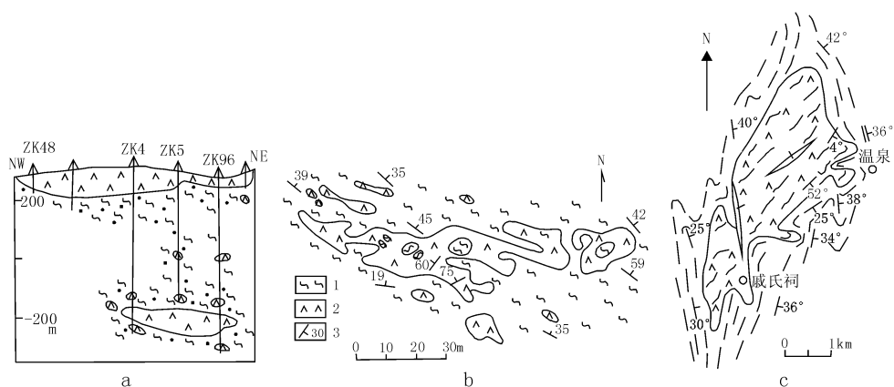
图4 较大无根超镁铁质岩块的剖面和平地质略图
