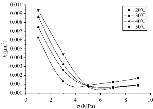
图 4 不同温度下铁法煤样渗透率随有效应力变化曲线 Fig 4 Changing curve of permeability for Tiefu coal at different temperatures
