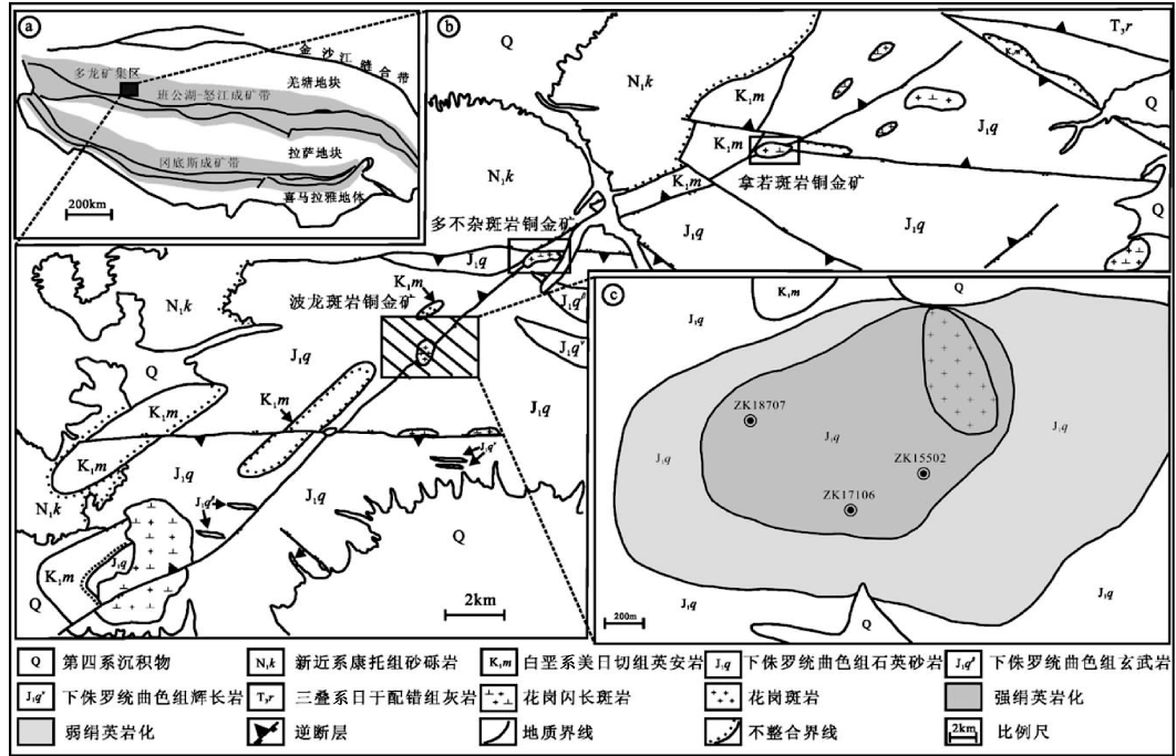
图 1 多龙矿集区构造背景简图 (a)、地质简图 (b) 和波龙矿床地质简图 (c) [4]
