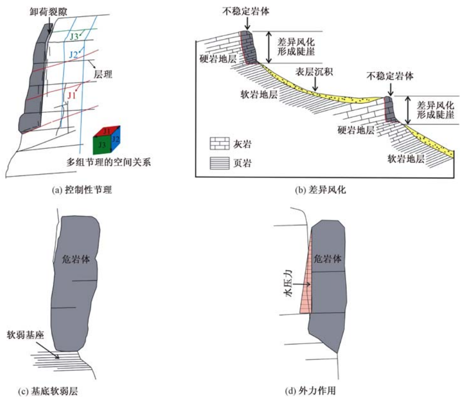
图 4 塔柱状岩体形成与失稳影响因素
