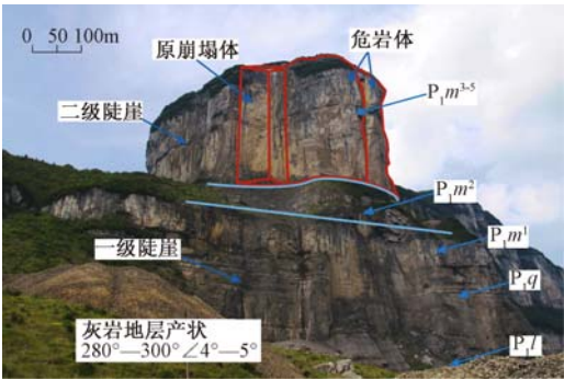
图 2 重庆市南川区甄子岩崩塌 Fig. 2 Zengziyan collapse in Nanchuan, Chongqing
