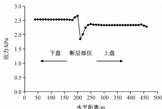
图6 沿高铁线路方向动应力分布曲线
