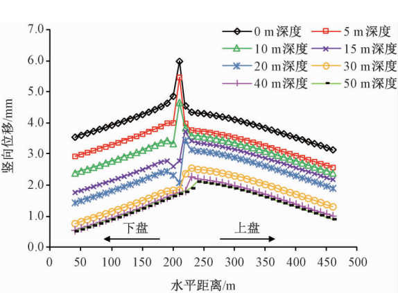
图13 列车动荷载与断层滑动共同作用所致竖向位移分布曲线
