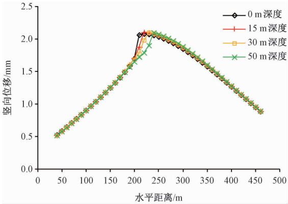
图11 断层滑动所致竖向位移分布曲线
