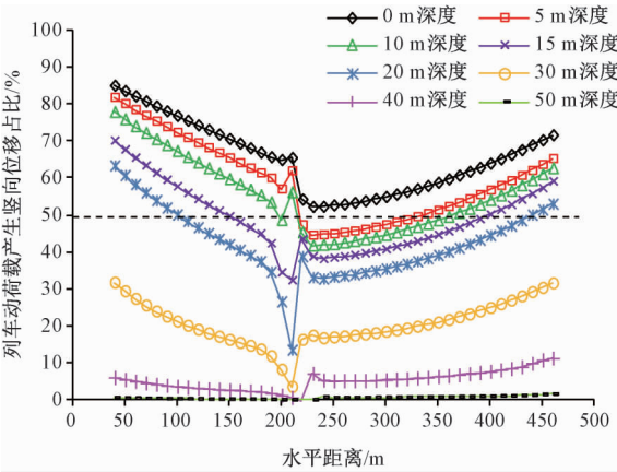
图14 列车动荷载产生竖向位移占总位移的百分比曲线
