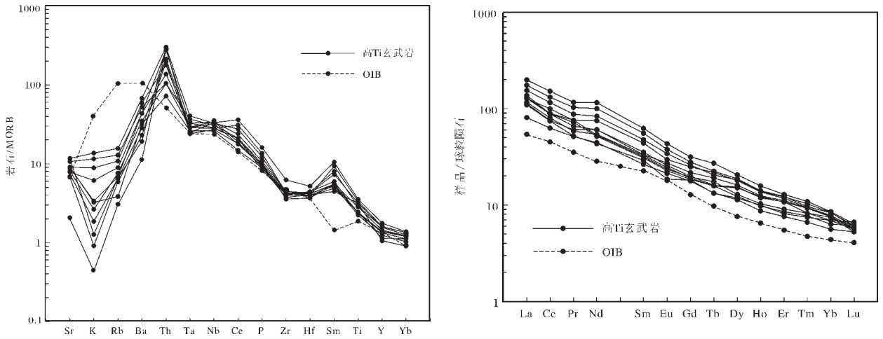
图3 当郎寨剖面杂岩组玄武岩微量元素蛛网图(左)和稀土元素配分型式(右)(标准化数值据参考文献[21])
