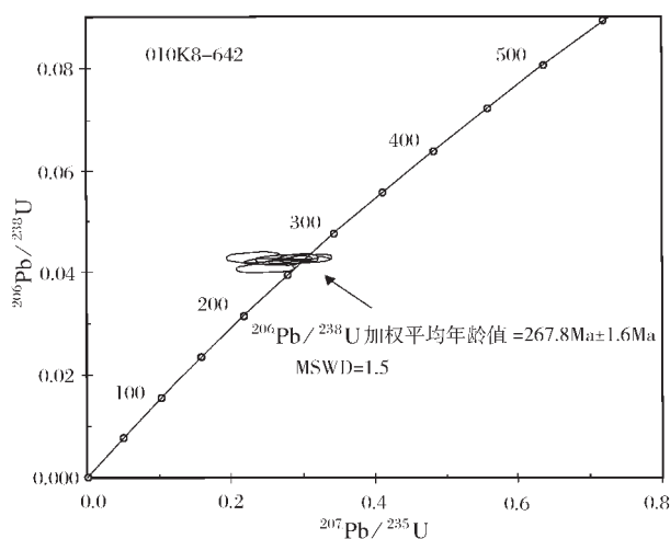
图3 石英闪长岩锆石SHRIMP U-Pb年龄谐和图
