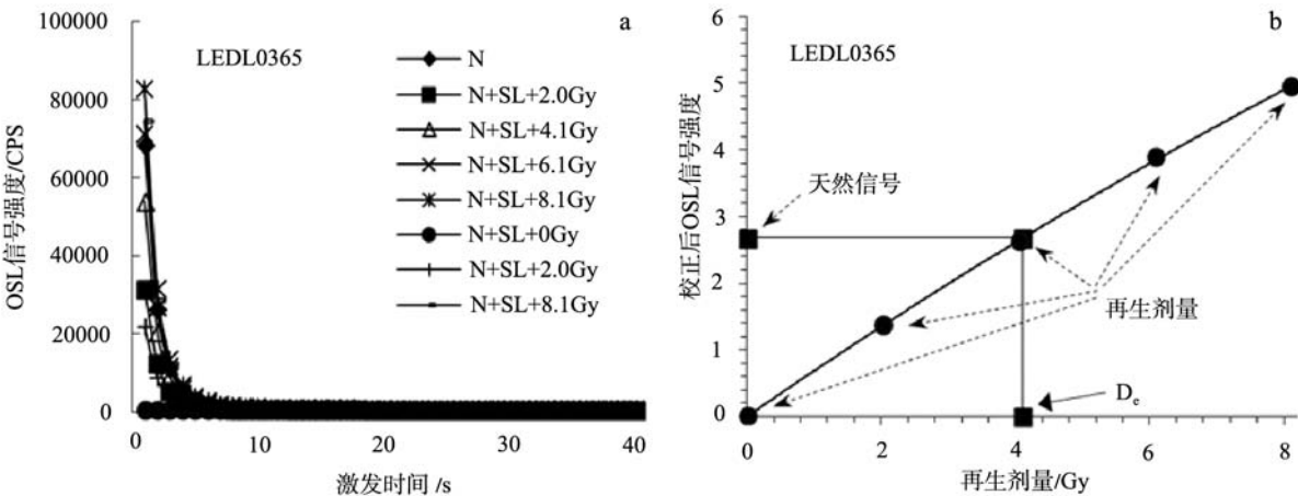
图 6 石英的 OSL 衰减曲线(a)和 SAR 再生剂量生长曲线(b) [67] Fig. 6 OSL signal decay curves (a) and SAR regenerated dose growth curve (b)
