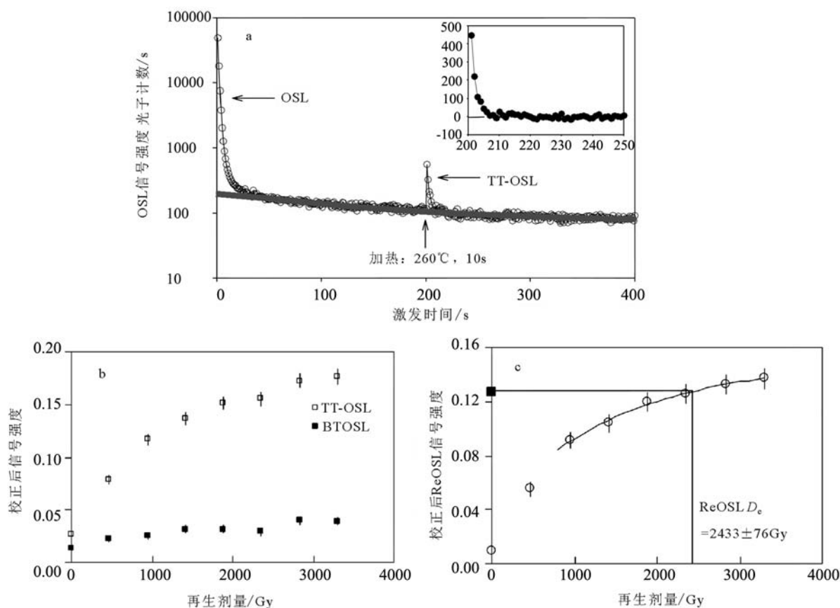
图8 蓝光晒退 200s 后加热 260°C、10s 所观察到的热转移光释光信号(a) [93] (嵌图为放大的减去慢速组分后的 TT-OSL 衰减曲线)、感量校正后的热转移光释光信号和基本转移光释光信号(b) [94] 和校正后回授光释光信号强度及 D_e 值测定(c) [94]
