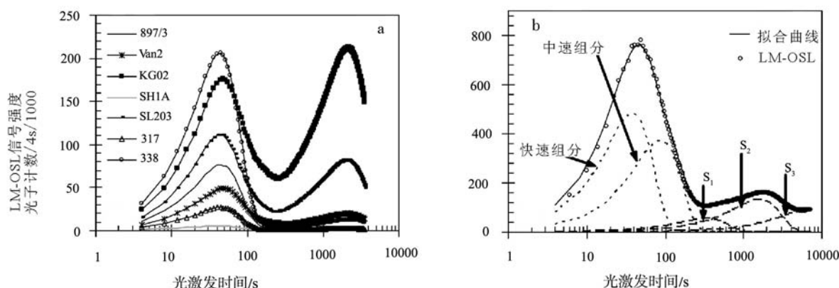
图5 来自不同地区石英样品7个的LM-OSL曲线(a) 与样品SL203的LM-OSL曲线(b) [46] (SL203样品为斯里兰卡沙丘沉积,约3.6ka)
