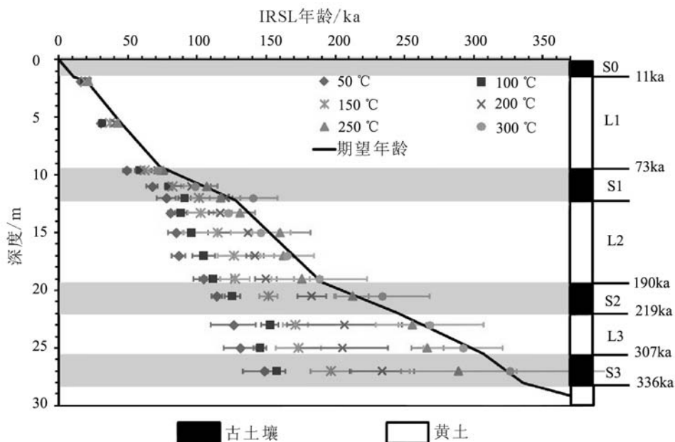
图10 MET-pIRIR 年龄与期望年龄及采样深度对比 [126]
