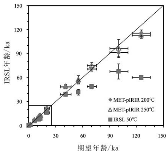
图9 长石在 50℃ 测量的 IRSL 年龄和使用 METpIRIR 法得到的 200℃ 和 250℃ 下 IRSL 年龄与根据石英 OSL 所获得的期望年龄或期望年龄比较 [20]
