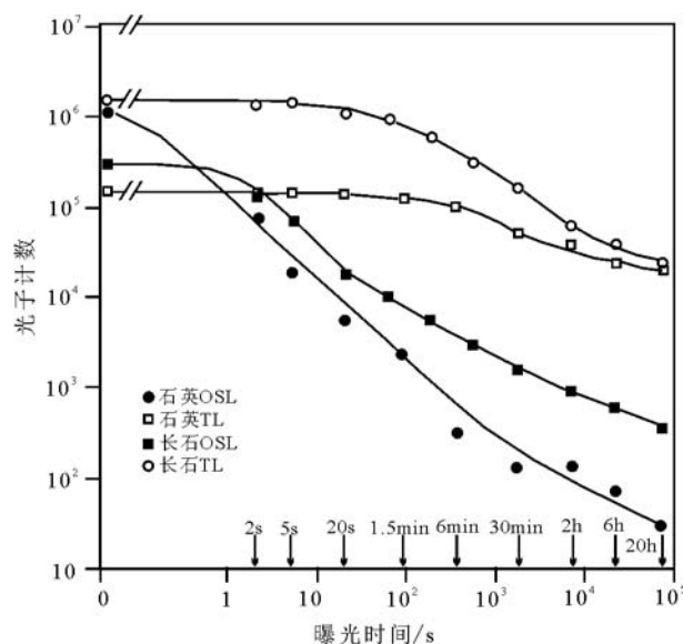
图4 石英与长石的光释光及热释光信号曝光效果 [8]
