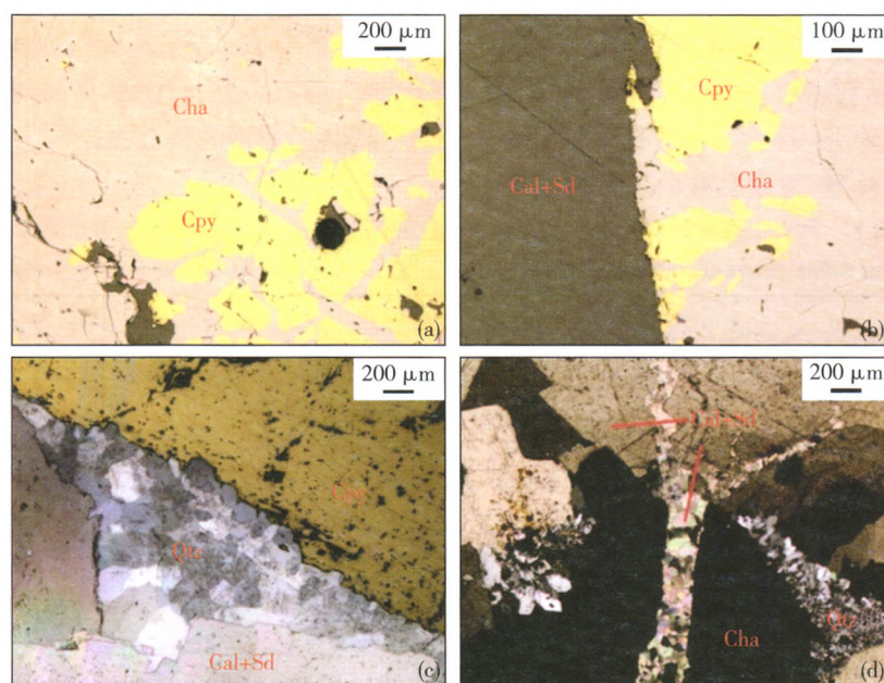
(a). 辉铜矿+黄铜矿脉(正交偏光);(b). 辉铜矿+黄铜矿+方解石+菱铁矿脉(正交偏光);(c). 黄铜矿+石英+方解石+菱铁矿脉(正交偏光);(d). 辉铜矿+石英+方解石+菱铁矿脉(正交偏光); Cha. 辉铜矿; Cpy. 黄铜矿; Cal. 方解石; Sd. 菱铁矿; Qtz. 石英。
