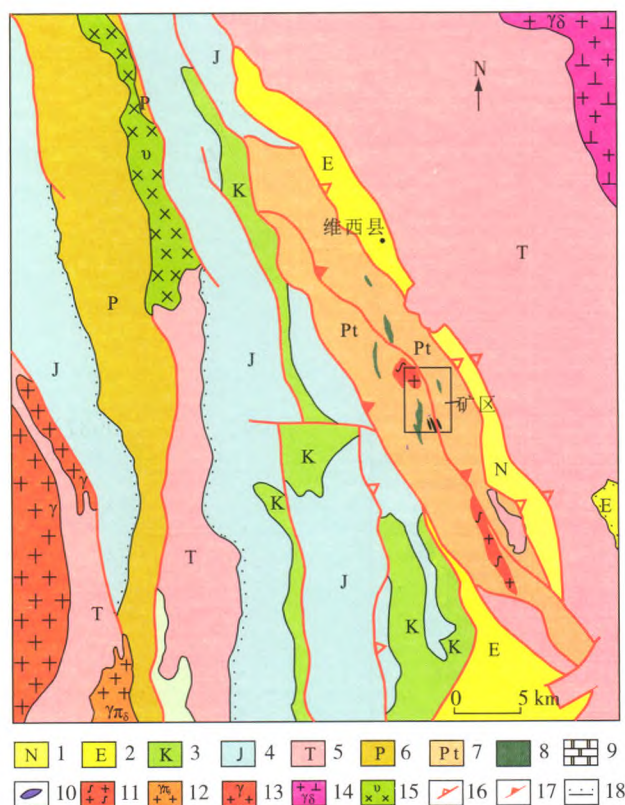
1. 新近系;2. 古近系;3. 白垩系;4. 侏罗系;5. 三叠系;6. 二叠系;7. 雪龙山岩群变质岩;8. 斜长角闪岩;9. 大理岩;10. 闪长岩脉;11. 花岗质糜棱岩;12. 喜山期花岗斑岩;13. 燕山期花岗岩;14. 印支期花岗闪长岩;15. 印支期辉长岩;16. 正断层;17. 逆断层;18. 不整合界线。
