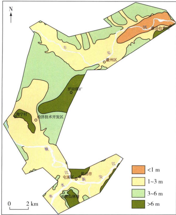
图 5 地下水位埋深分布图 Fig. 5 Map showing distribution of water tables
