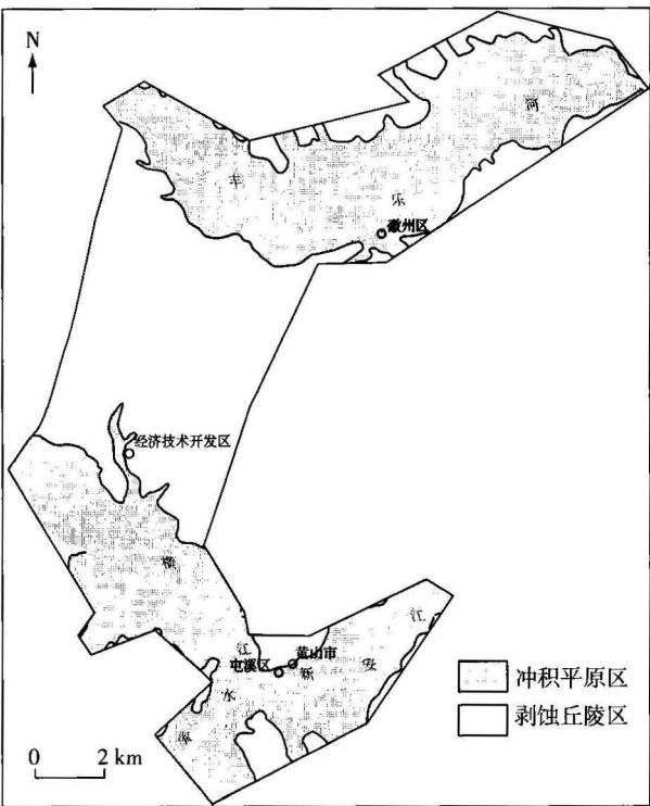
图 4 工程地质分区图 Fig. 4 Map showing the engineering geological division
