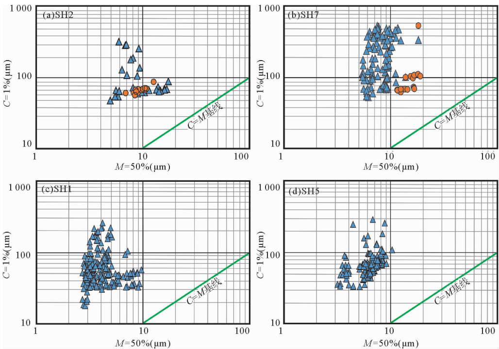
图 5 神狐海域 GMGS01 区块 SH2、SH7、SH1 和 SH5 站位的粒度 C-M 图版 Fig. 5 Grain size C-M pattern at sites SH2, SH7, SH1 and SH5 in GMGS01 of the Shenhu Area
