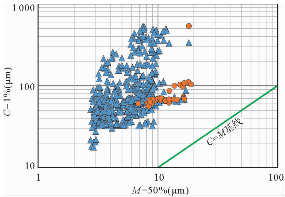
图 6 神狐海域 GMGS01 区块粒度 C-M 综合图版 (利用 SH2、SH7、SH1 和 SH5 站位)
