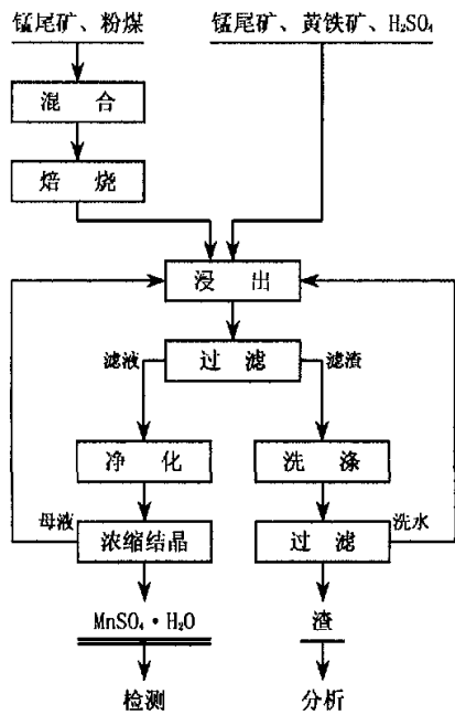
图 1 锰尾矿回收锰试验流程
