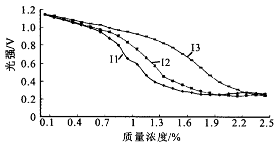
图2 不同光源功率条件下散射特性曲线
