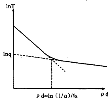
图4 散射总强度对数
