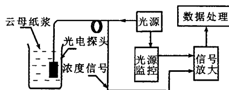
图1 浓度测试仪系统结构
