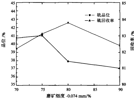
图2 硫粗选磨矿细度实验结果
