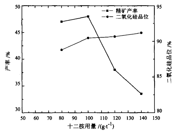
图 6 十二胺用量实验结果 Fig. 6 Test results of dodecamine dosage
