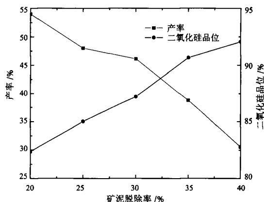
图5 脱泥实验结果
