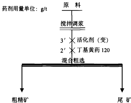
图1 硫粗选活化剂探索实验工艺流程及条件
