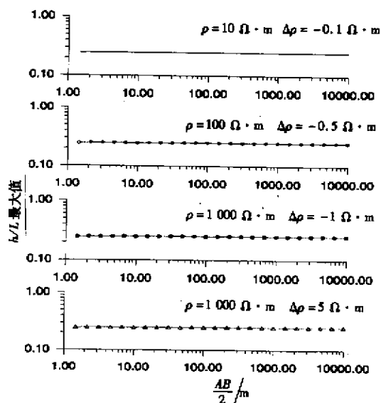
图 2 最大灵敏度处 h/L 随供电电极距 L 变化曲线
