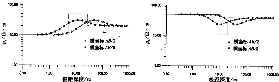
图 3 三层电阻率曲线与真实模型对比
