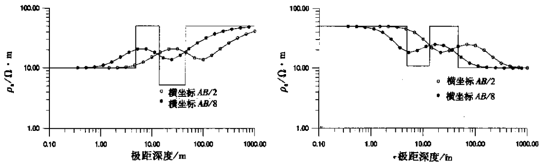
图4 四层电阻率曲线与真实模型对比
