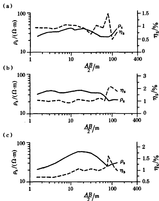
图 3 激电测深 \rho_s 及 \eta_s 曲线
