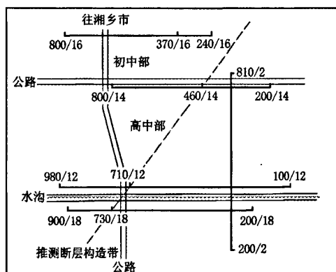
图 1 东山学校水文物探测线布置示意
