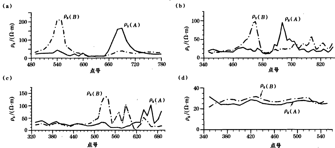
图 2 联合剖面法 \rho_s 曲线
