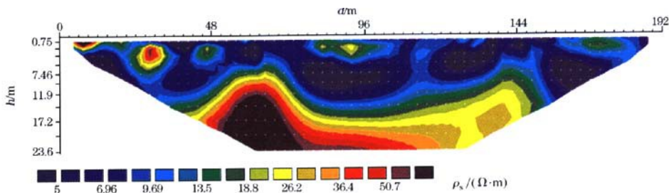
图 1 L3 线高密度反演效果
