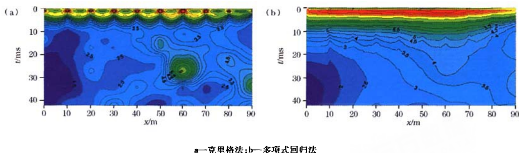
图3 L5线 \rho_s 等值线不同网格化方法结果对比
