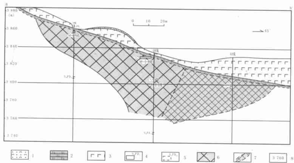
图 3 雪泉洞 ( 锌 ) 号沟铜矿体矿形态示意图 ( 据扬合群, 2001)
