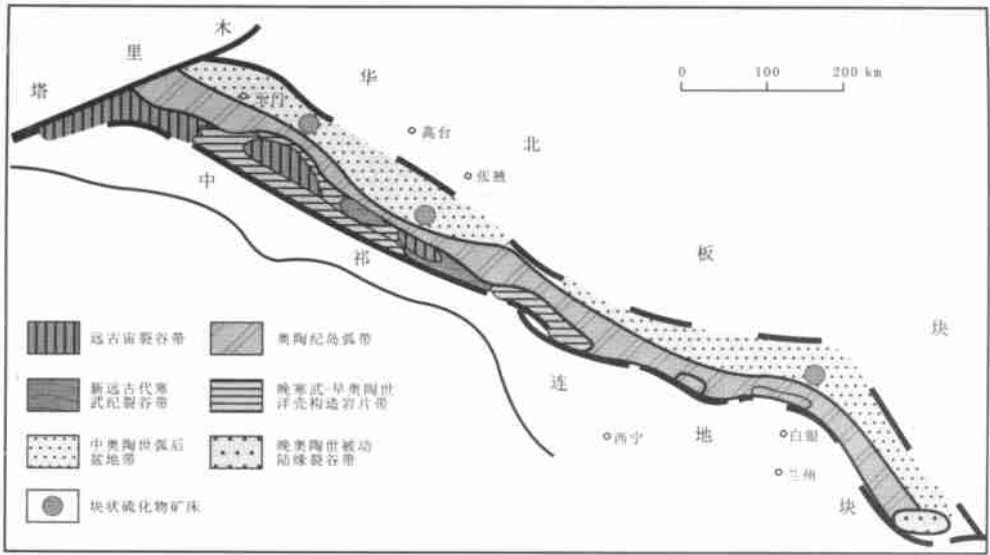
图 1 北祁连山区域构造略图（据夏林圻等，2001） Fig. 1 Geological sketch map of north Qilian mountains
