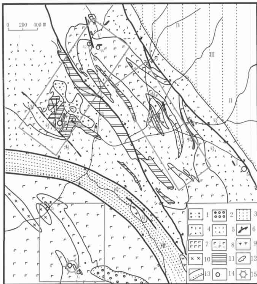
图 2 雪泉铜(锌)矿床地质草图
