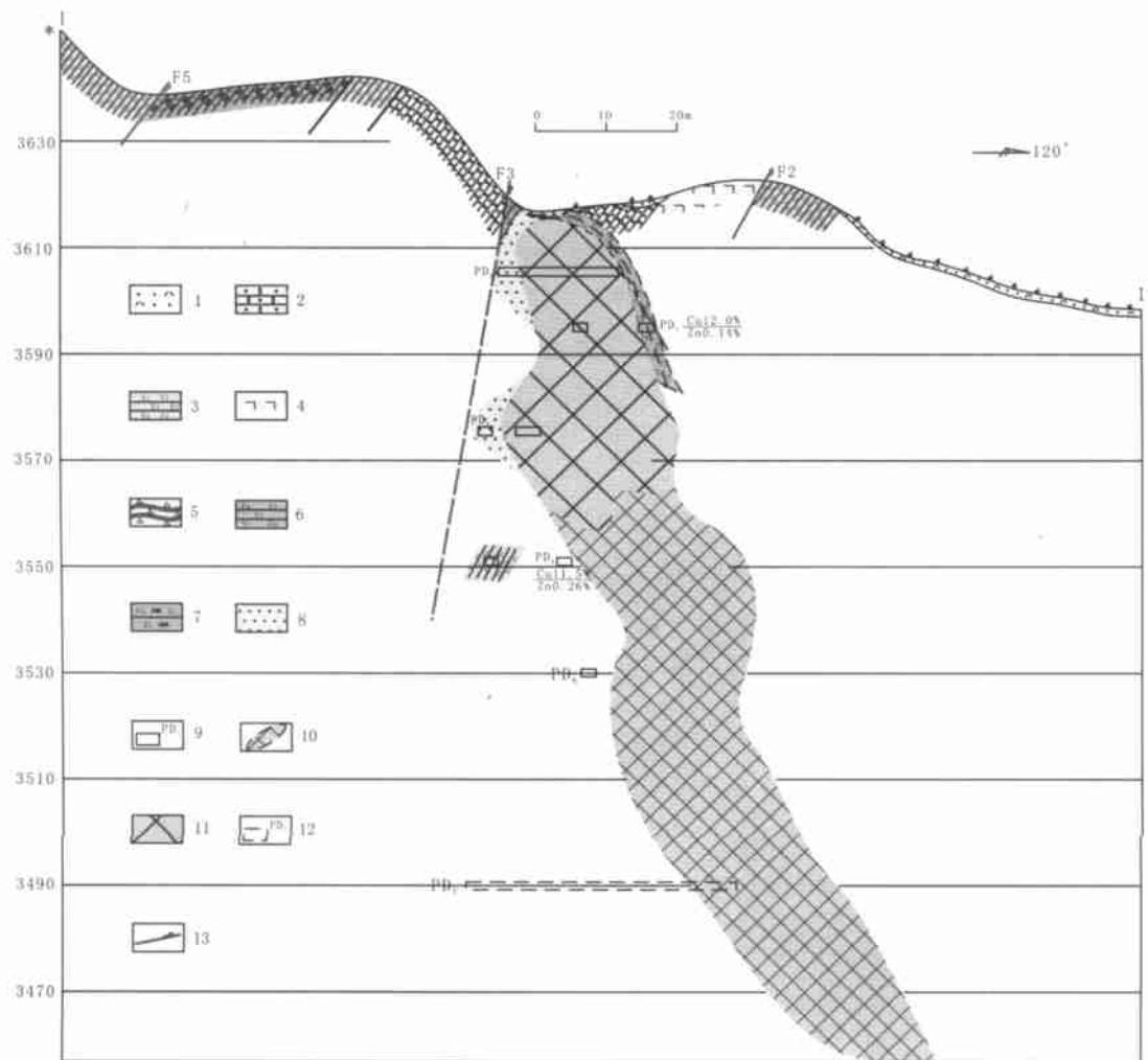
图 4 雪泉铜 ( 锌 ) 矿北矿段铜矿体横剖面投影图
