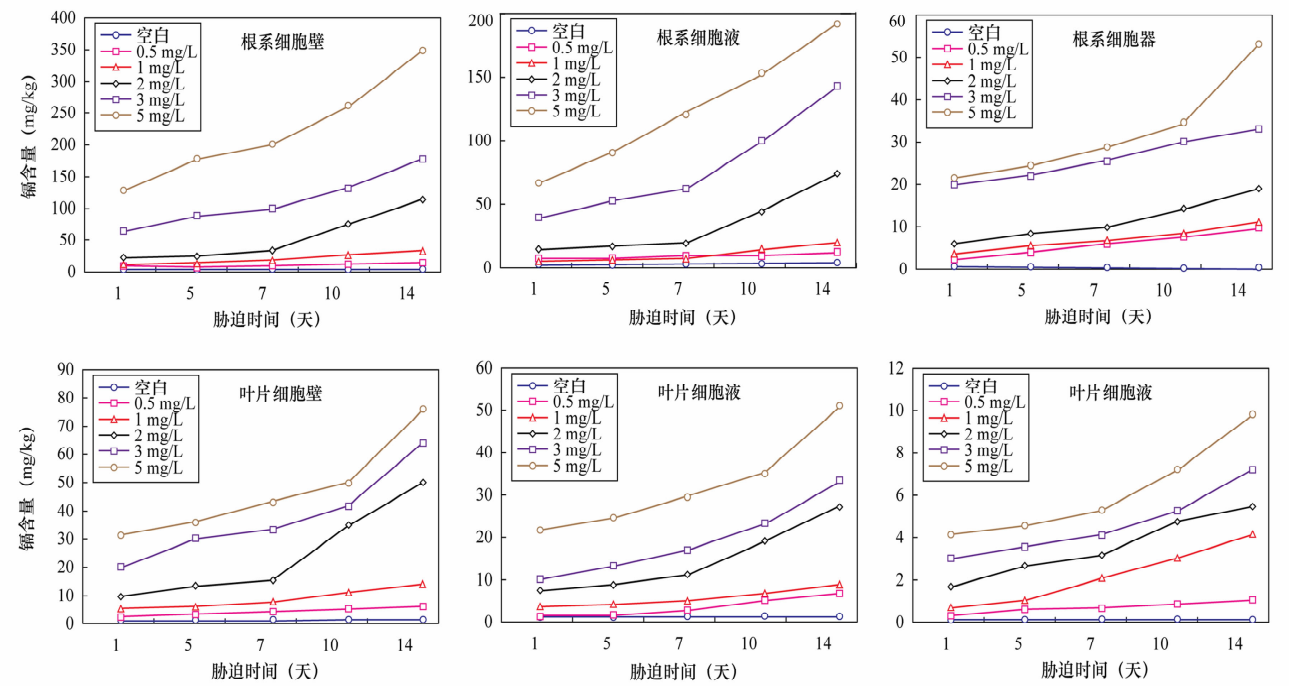
图 2 不同镉刺激浓度和时间下根系和叶片细胞中镉含量分布规律 Fig. 2 Subcellular distribution of cadmium in root and leaf samples
