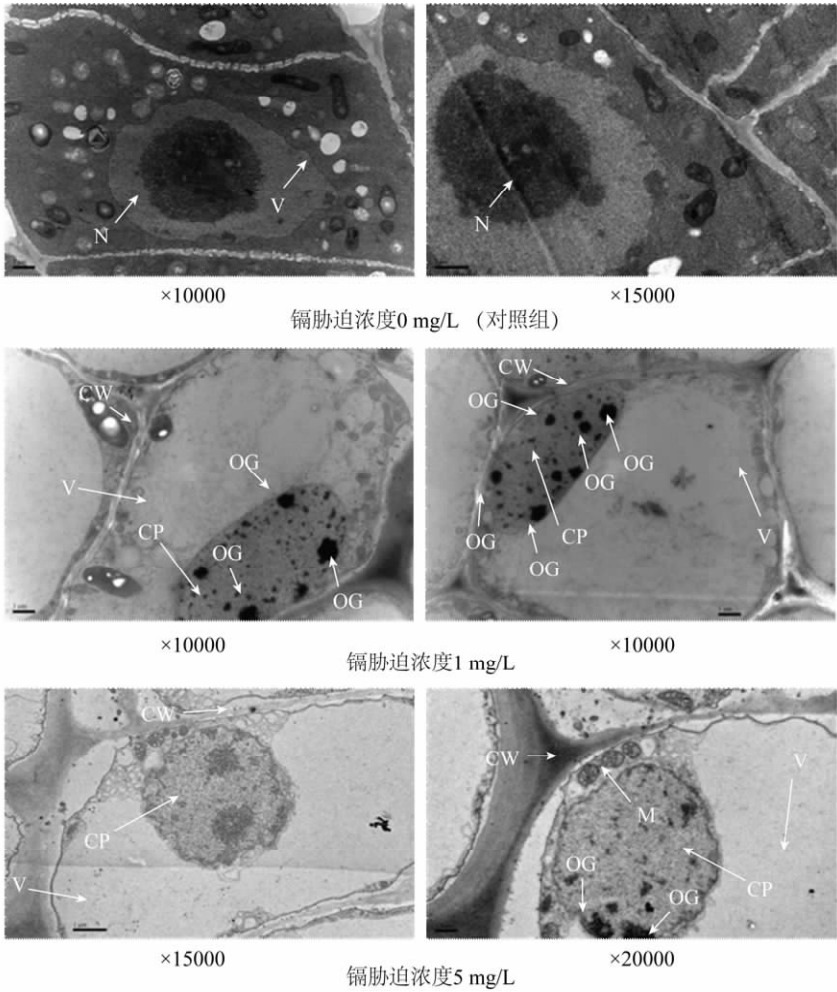
图 3 不同镉浓度下印度芥菜根系的显微结构 Fig. 3 SEM maps of subcellular under different cadmium disposal in root samples Chl—叶绿体;CP—细胞质;V—液泡;CW—细胞壁;M—线粒体;PM—细胞质膜;SG—淀粉粒;OG—嗜饿颗粒;N—细胞核。
